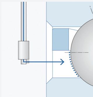
平行ノズル
