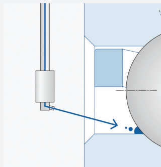
斜めノズル
