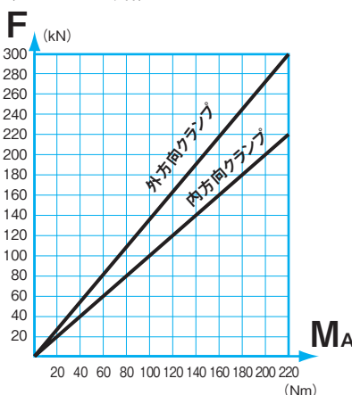
クランプ力と締付トルク(SW2)の関係 (MPSD-120の場合)
