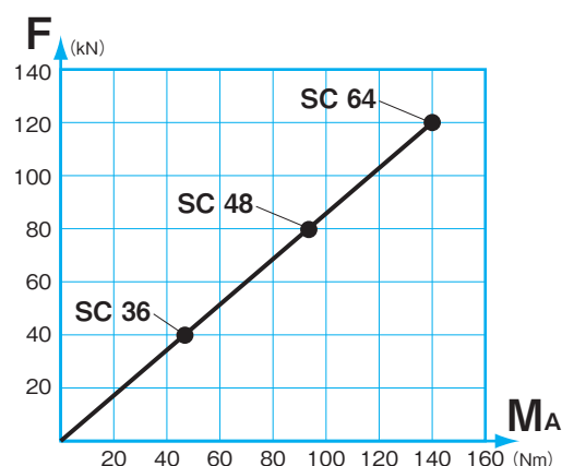
トルクとクランプ力の関係
