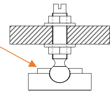
オプション Retaining clips
