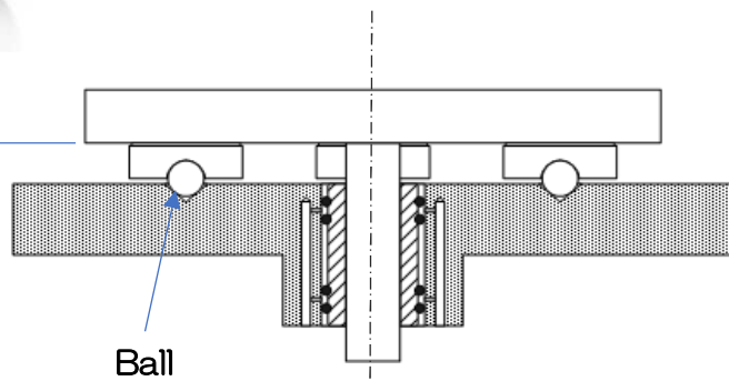
ロータリーテーブルでの使用例
