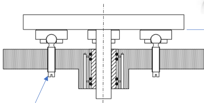
Round Endタイプ
