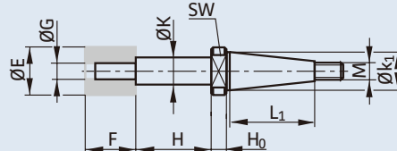
図2 ねじで砥石を取付け(PS)
