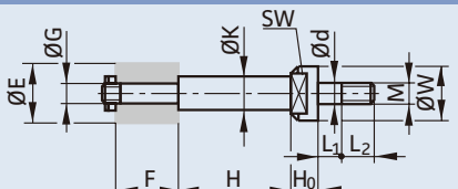
図4 ナットで砥石を取付け(MU)
