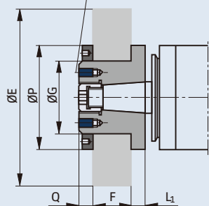
図3 フランジ形状 SN
