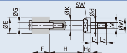
図2 ねじで砥石を取付け(PS)
