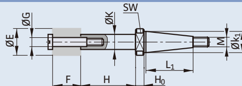
図2 ねじで砥石を取付け(PS)
