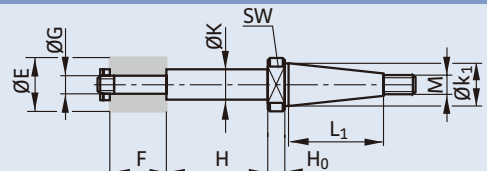
図4 ナットで砥石を取付け(MU)
