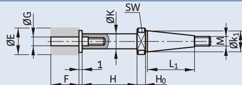
図3 スタッドボルトで砥石を取付け(PS)
