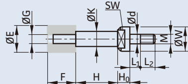
図2 ねじで砥石を取付け(PS)
