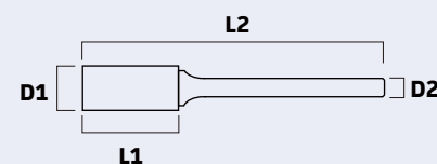
3mm シャンクダブルカット (オール超硬)
