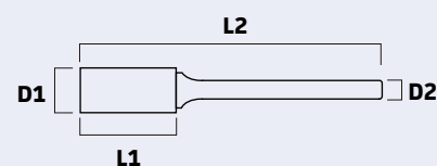
3mm シャンクダブルカット (オール超硬)
