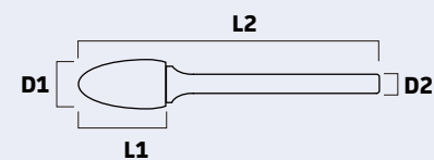
3mm シャンクシングルカット (オール超硬)
