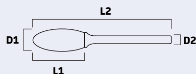
3mm シャンクシングルカット (オール超硬)
