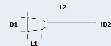
3mm シャンクシングルカット(オール超硬)
