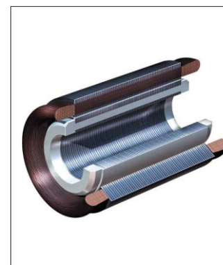
■モータエレメント
