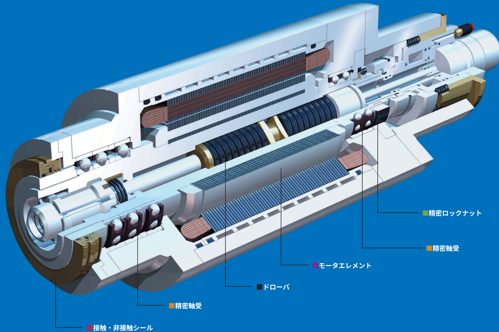
■接触・非接触シール
