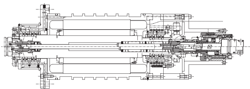
マシニングセンタ用スピンドル 回転数：10000min -1 潤滑：オイルミスト潤滑
