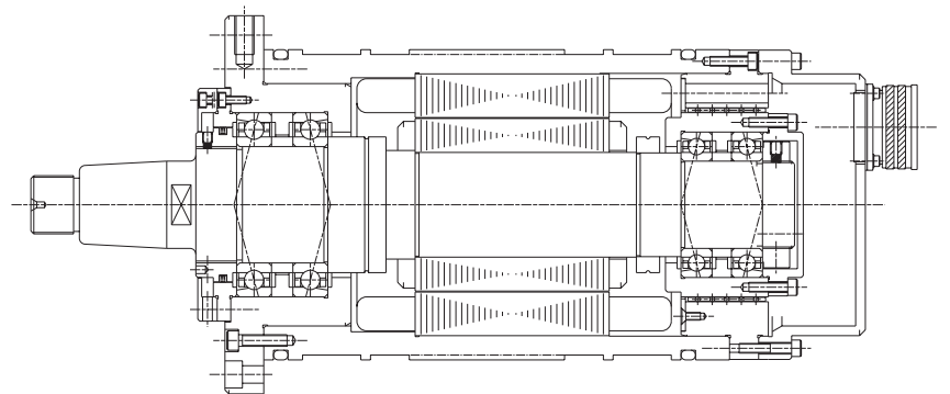
研削用スピンドル 回転数：3000min -1 潤滑：グリース潤滑
