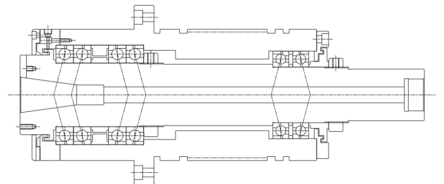
ミーリング用スピンドル 回転数：3000min -1 潤滑：グリース潤滑
