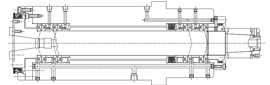
ミーリング用スピンドル 回転数：15000min -1 潤滑：オイルミスト潤滑
