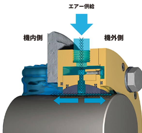
エアの流れ
