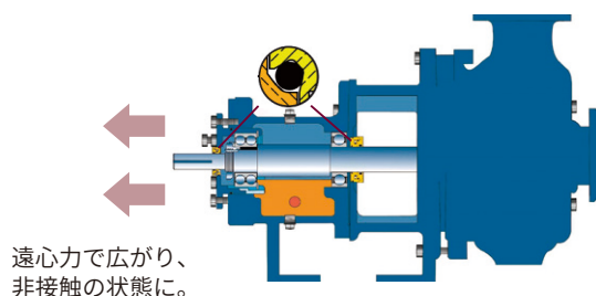
運転時（軸受箱：内圧上昇）
