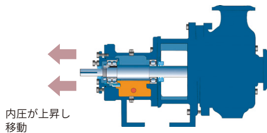
運転時（軸受箱：内圧上昇）
